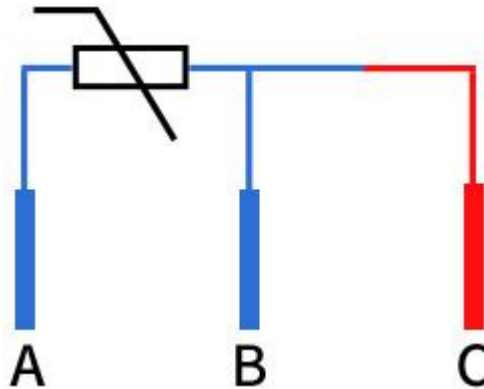
PT100 传感器
